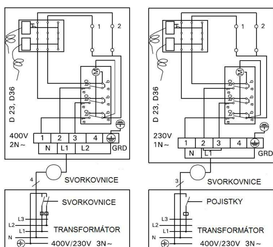
Obr. 10 Elektrické zapojení kamen (D23, D36)
